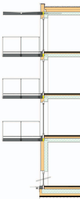
Fassadenschnitt
